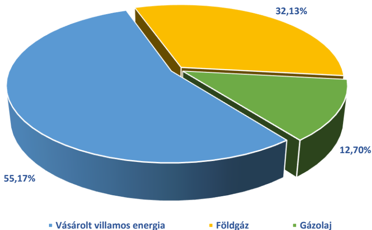
ENERGIAMÉRLEG [MWhpr/év] PALCSÓ ZOLTÁN KERESKEDELMI KFT összesen 2022.
